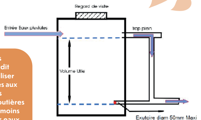
Schéma de principe d'une cuve de rétention/régulation.
